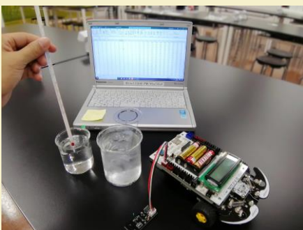
温度センサーを使った実験
